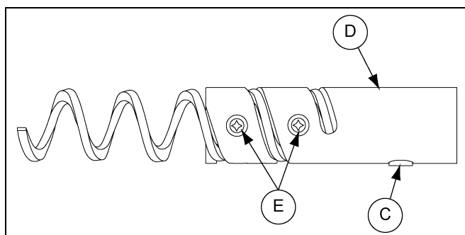
Рисунок 5AL Каплеуловитель Соединение с драйвером модели 220
