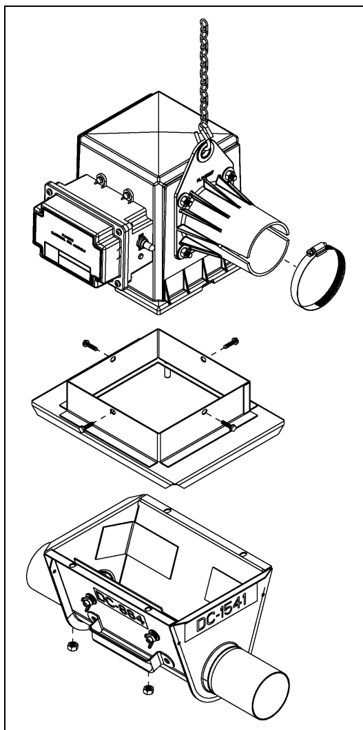
Рисунок 5AJ Загрузочный бункер
