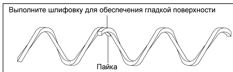
Рисунок 5AI Пайка шнека
