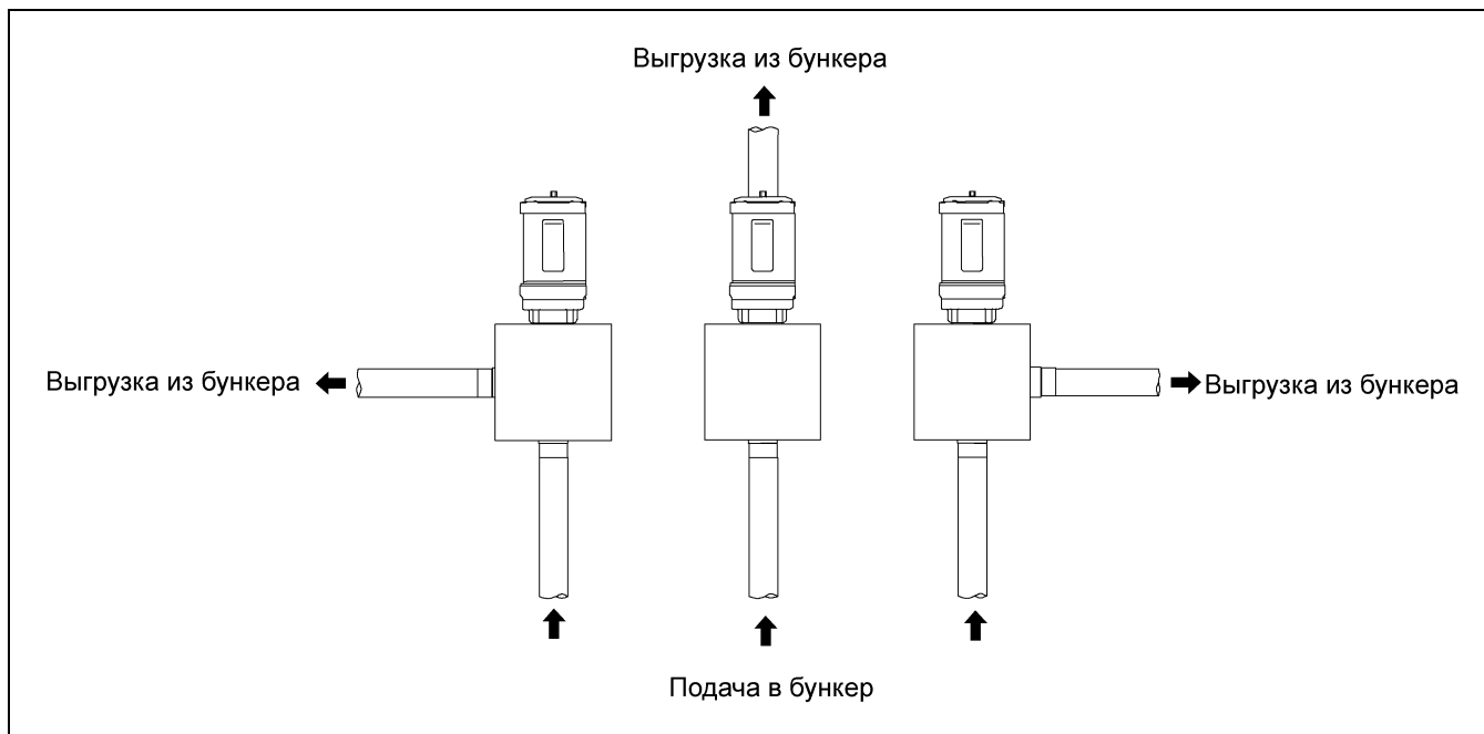
Рисунок 5АО Направления установки воронки
