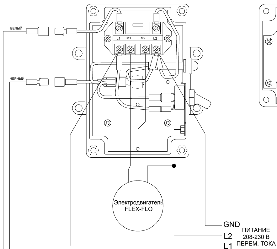
СИСТЕМА ЗАПОЛНЕНИЯ БЛОКА УПРАВЛЕНИЯ FLEX-FLO (FLX-4512)
