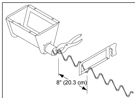
Рисунок 5AH Обрезка шнека
