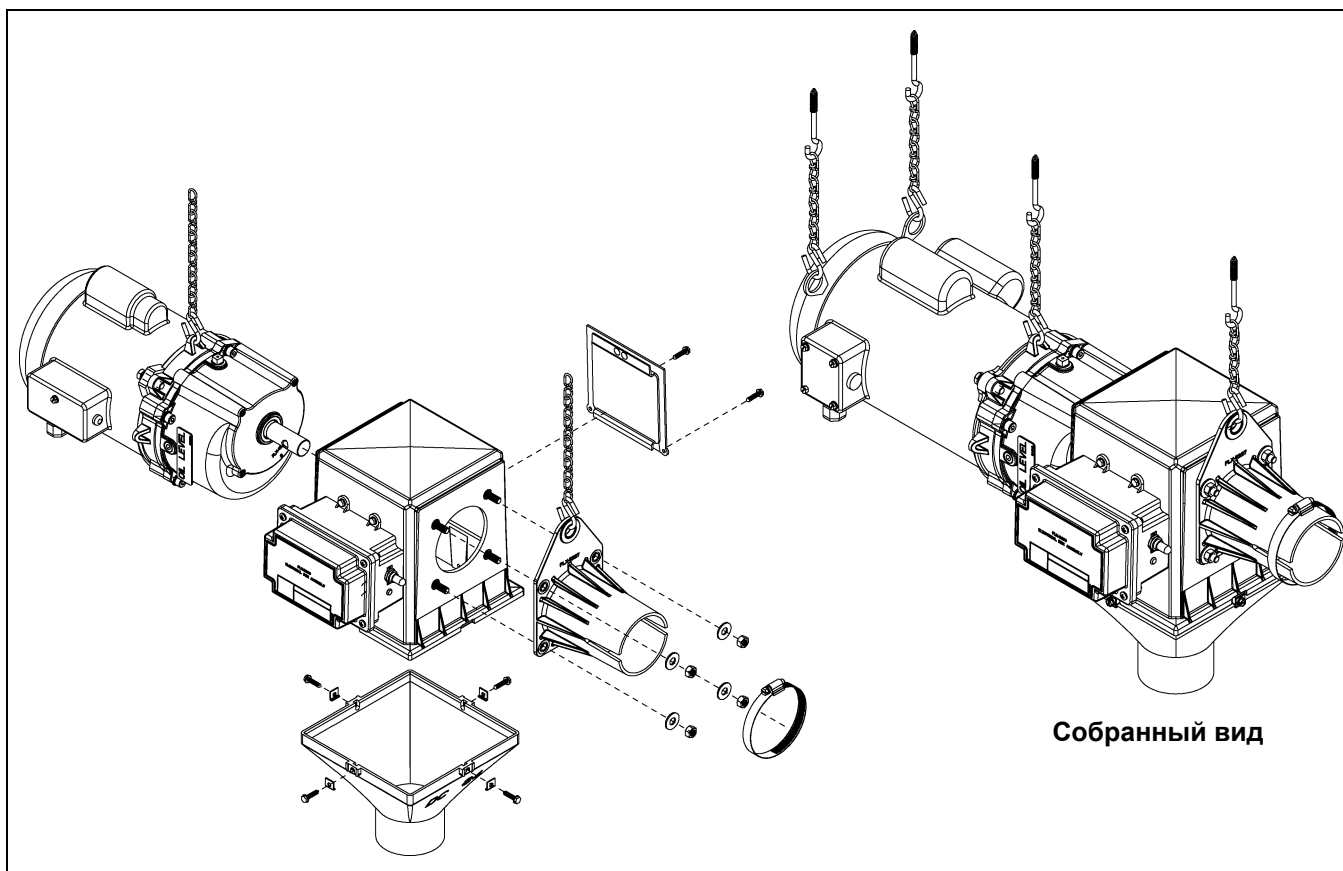
Рисунок 5Z Прямой привод/двигатель
