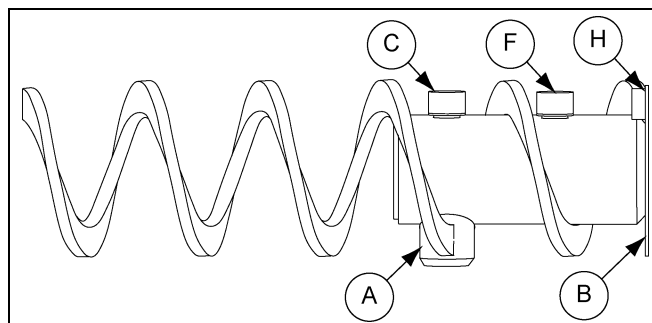
Рисунок 5AM Соединение с драйвером модели 300/модели 350
