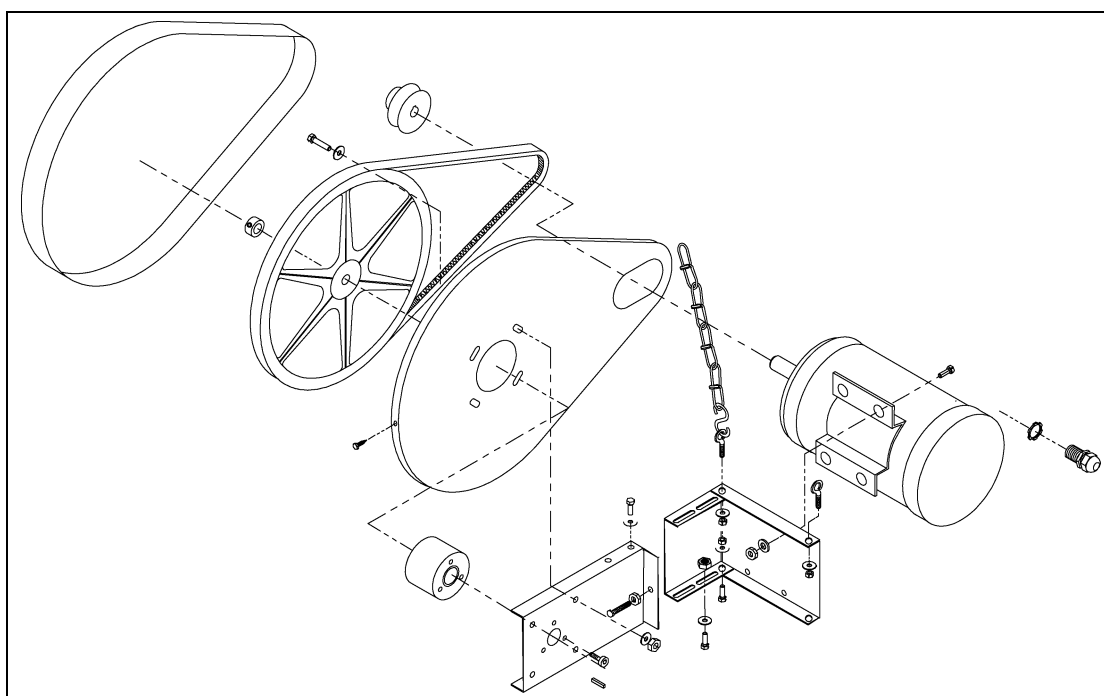
Рисунок 5AE Ременный привод/двигатель
